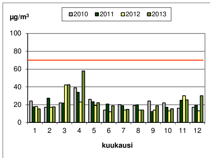
Kuva 49. Hengitettävien hiukkasten ohjearvoon ( 70 \mu\text{g}/\text{m}^3 ) verrattavat vuorokausikeskiarvot Naantalissa vuosina 2010 - 2013.
