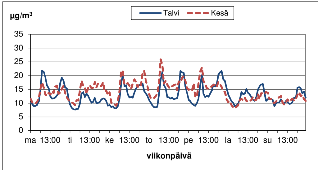
Kuva 39. Raision hengitettävien hiukkasten pitoisuuden vaihtelut viikon eri ajankohtina kesällä (1.4.–30.9.) ja talvella (1.1.–31.3. ja 1.10.–31.12.) vuonna 2013.
