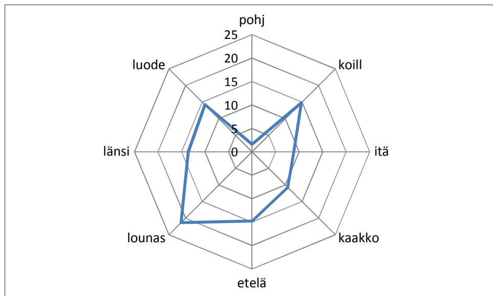
Kuva 4. Tuulensuunnan jakautuminen Turun Juhannuskukkulalla vuonna 2013.
