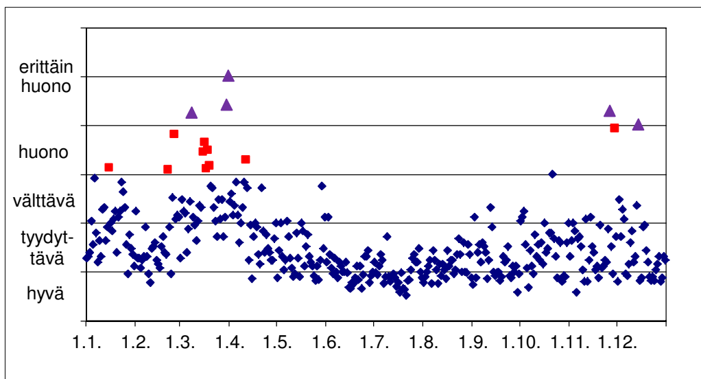
Kuva 7. Turun keskustan ilmanlaatu indeksillä kuvattuna vuonna 2013.
