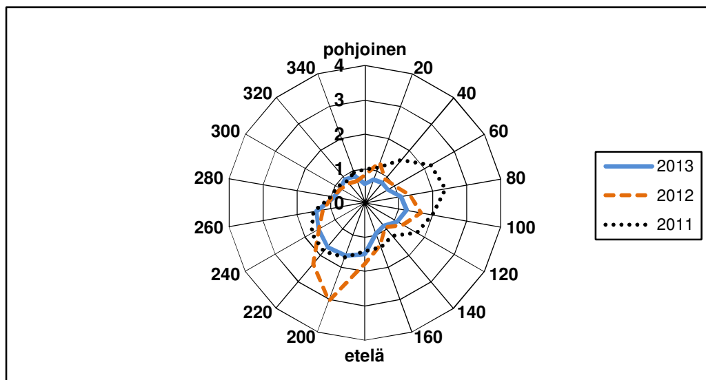
Kuva 32. Kaanaan rikkidioksidin keskipitoisuus (µg/m 3 ) eri tuulen suunnilla vuosina 2011, 2012 ja 2013.
