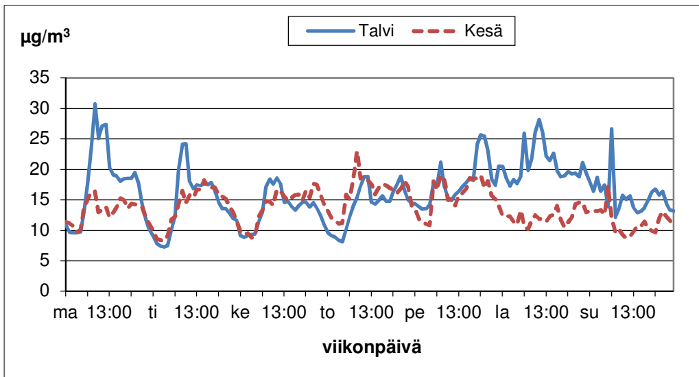
Kuva 22. Kauppatorin hengitettävien hiukkasten pitoisuuden vaihtelut viikon eri ajankohtina kesällä (1.4.–30.9.) ja talvella (1.1.–31.3. ja 1.10.–31.12.) vuonna 2013.
