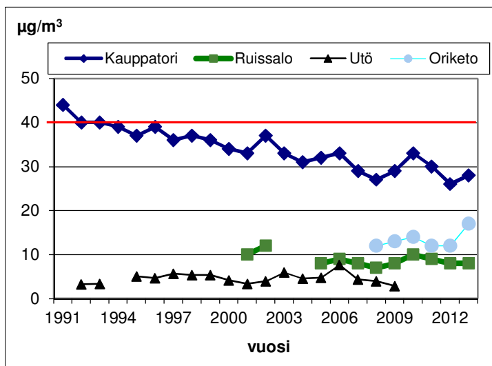
Kuva 12. Typpidioksidipitoisuuden vuosikeskiarvot Turun Kauppatorilla, Ruissalossa ja Utössä. Orikedolla mittaukset aloitettiin helmikuussa 2008.
