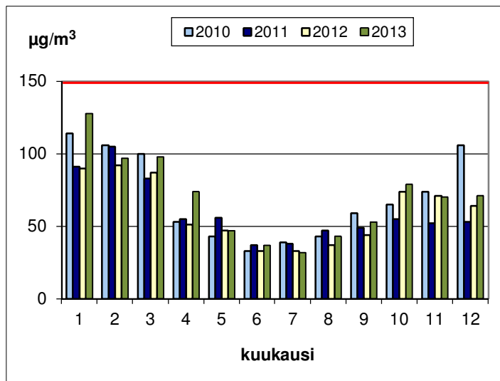
Kuva 35. Typpidioksidin ohjearvoon verrattavat tuntikeskiarvot Raisiossa vuosina 2010 - 2013.
