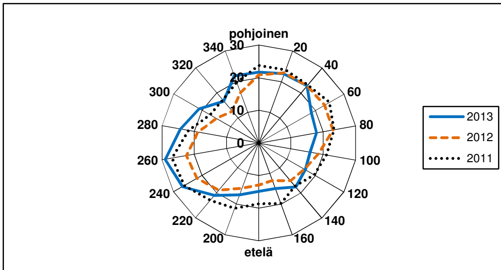
Kuva 37. Raision typpidioksidin keskipitoisuus ( \mu\text{g}/\text{m}^3 ) eri tuulen suunnilla vuosina 2011, 2012 ja 2013.
