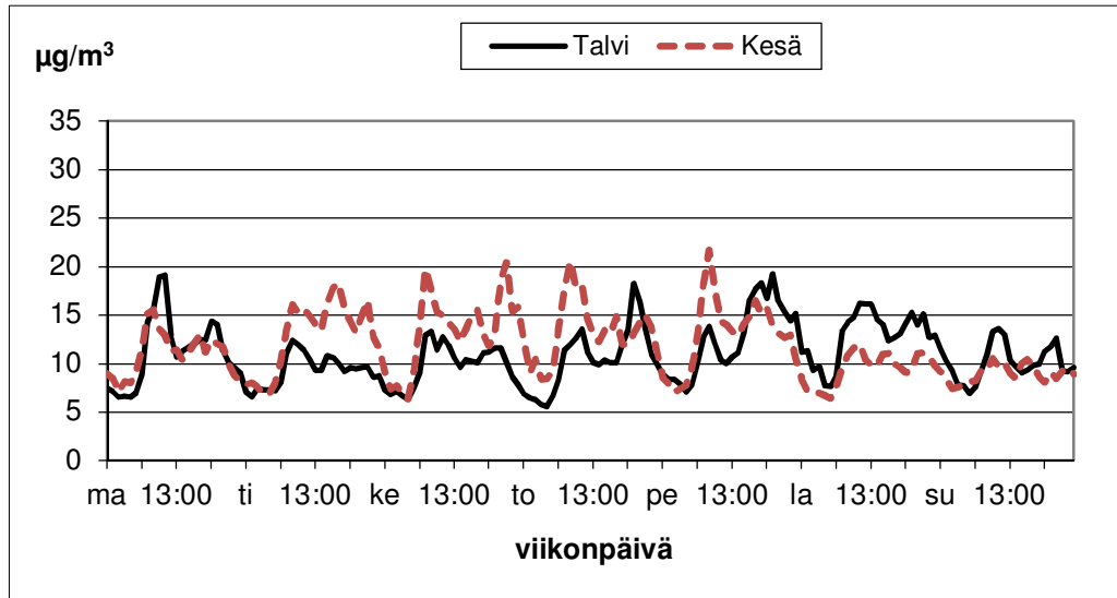
Kuva 50. Naantalin hengitettävien hiukkasten pitoisuuksien vaihtelut viikon eri ajankohtina kesällä (1.4.–30.9.) ja talvella (1.1.–31.3. ja 1.10.–31.12.) vuonna 2013.
