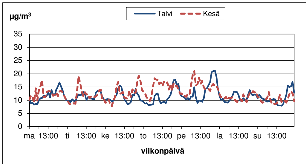
Kuva 60. Paraisten hengitettävien hiukkasten pitoisuuksien vaihtelut viikon eri ajankohtina kesällä (1.4.–30.9.) ja talvella (1.1.–31.3. ja 1.10.–31.12.) vuonna 2013.
