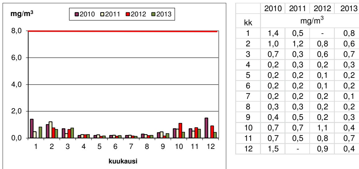
Kuva 24. Hiilimonoksidin ohjearvoon ( 8 \text{ mg/m}^3 ) verrattavat 8 tunnin keskiarvot Kauppatorilla vuosina 2010 - 2013. Joulukuun 2011 ja tammikuun 2012 tulokset puuttuvat laitevian vuoksi.
