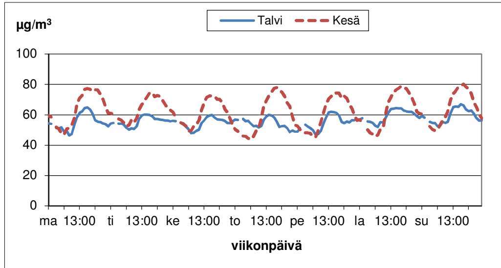
Kuva 28. Ruissalon otsonipitoisuuden vaihtelut viikon eri ajankohtina kesällä (1.4.–30.9.) ja talvella (1.1.–31.3. ja 1.10.–31.12.) vuonna 2013.
