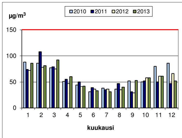
Kuva 46. Typpidioksidin ohjearvoon verrattavat tuntikeskiarvot Naantalissa vuosina 2010 - 2013. Heinäkuussa 2010 mittausten ajallinen kattavuus oli vain 85 %.
