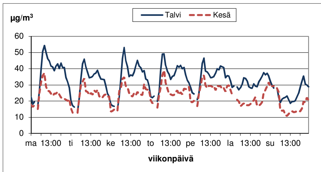
Kuva 17. Kauppatorin typpidioksidipitoisuuden vaihtelut viikon eri ajankohtina kesällä (1.4.–30.9.) ja talvella (1.1.–31.3. ja 1.10.–31.12.) vuonna 2013.
