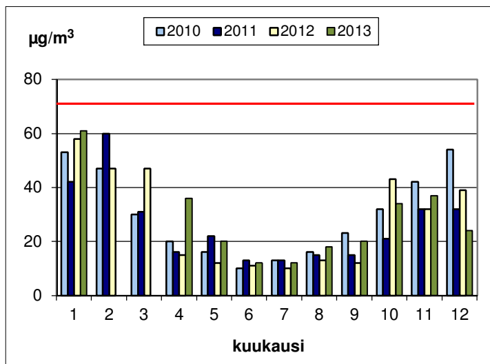
Kuva 52. Typpidioksidipitoisuuden ohjearvoon verrattavat vuorokausikeskiarvot Kaarinassa vuosina 2010 - 2013. Huhtikuussa 2010 tulosten ajallinen kattavuus oli vain 78 %, tammikuussa 2012 86 % ja syyskuussa 2012 84 %. Helmi- ja maaliskuun 2013 tulokset puuttuvat laitevian vuoksi.
