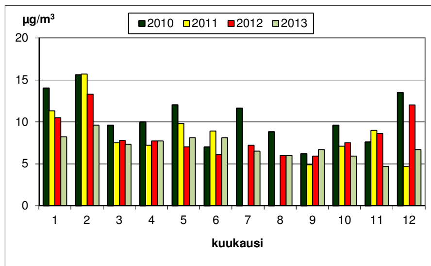
Kuva 21. Oriekedon pienhiukkaspitoisuuden ( PM_{2,5} ) kuukausikeskiarvot vuosina 2010 - 2013. Heinä- ja elokuu 2011 puuttuvat laitevian vuoksi.
