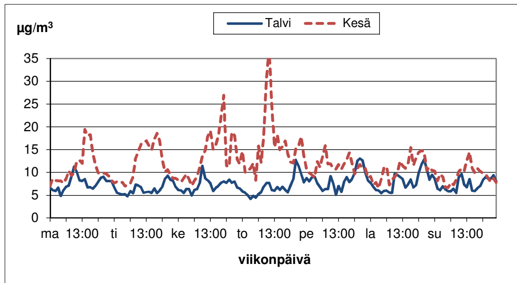
Kuva 57. Kaarinan hengitettävien hiukkasten pitoisuuksien vaihtelut viikon eri ajankohtina kesällä (1.4.–30.9.) ja talvella (1.1.–31.3. ja 1.10.–31.12.) vuonna 2013.
