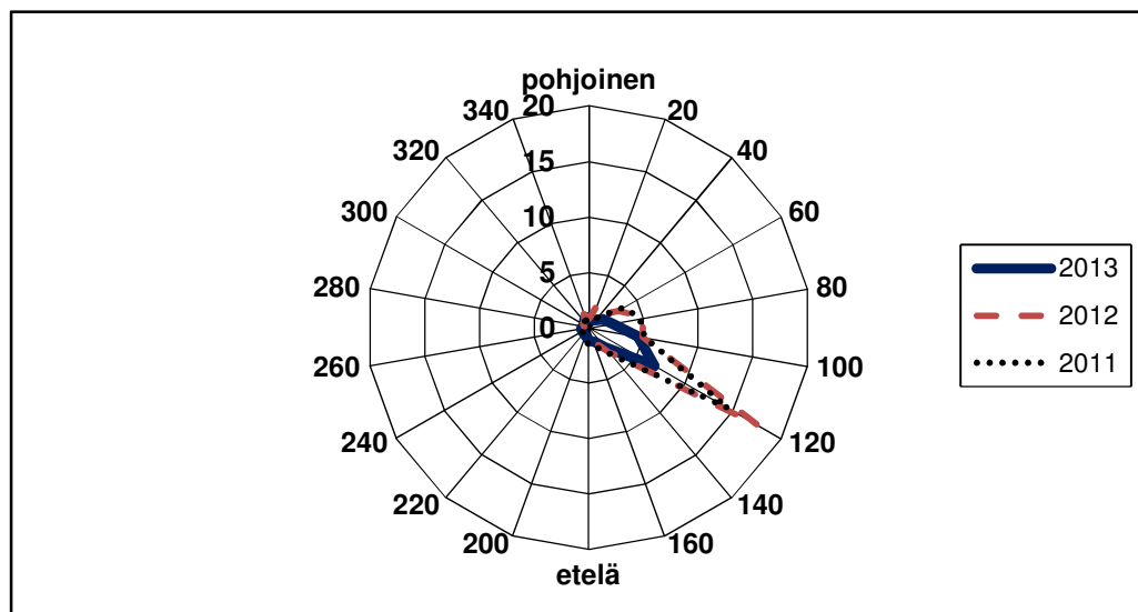
Kuva 43. Naantalin rikkidioksidin keskipitoisuus (µg/m 3 ) eri tuulen suunnilla vuosina 2011, 2012 ja 2013.
