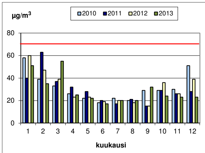
Kuva 45. Typpidioksidipitoisuuden ohjearvoon verrattavat vuorokausikeskiarvot Naantalissa vuosina 2010 – 2013. Heinäkuussa 2010 mittausten ajallinen kattavuus oli vain 85 %.
