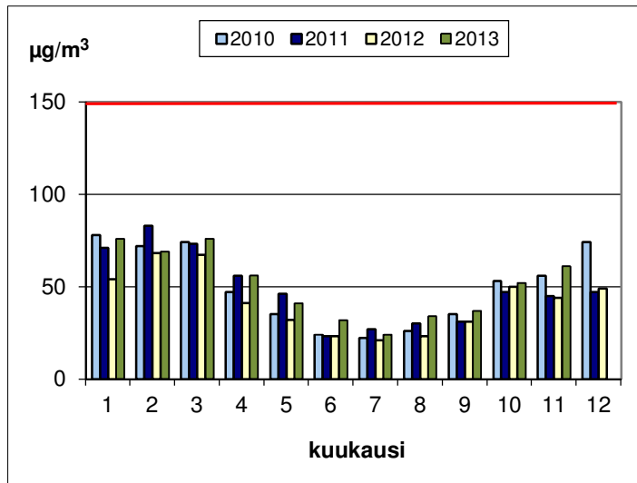
Kuva 16. Typpidioksidipitoisuuden ohjearvoon verrattavat tuntikeskiarvot Turun Orikedolla vuosina 2010 – 2013. Toukokuussa 2010 mittausten ajallinen kattavuus oli vain 81 %, kesäkuussa 2012 77 % ja heinäkuussa 87 %. Joulukuun 2013 ohjearvovertailu puuttuu laitevian vuoksi.
