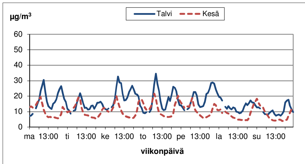
Kuva 54. Kaarinan typpidioksidipitoisuuden vaihtelut viikon eri ajankohtina kesällä (1.4.–30.9.) ja talvella (1.1.–31.3. ja 1.10.–31.12.) vuonna 2013.
