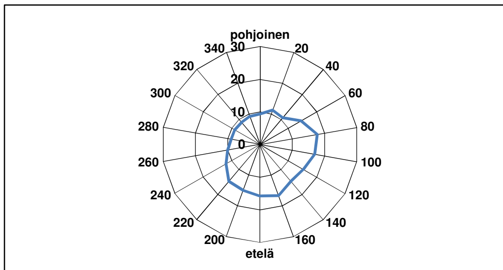
Kuva 61. Paraisten hengitettävien hiukkasten keskipitoisuus ( \mu\text{g}/\text{m}^3 ) eri tuulen suunnilla 2.3.–31.12.2013.
