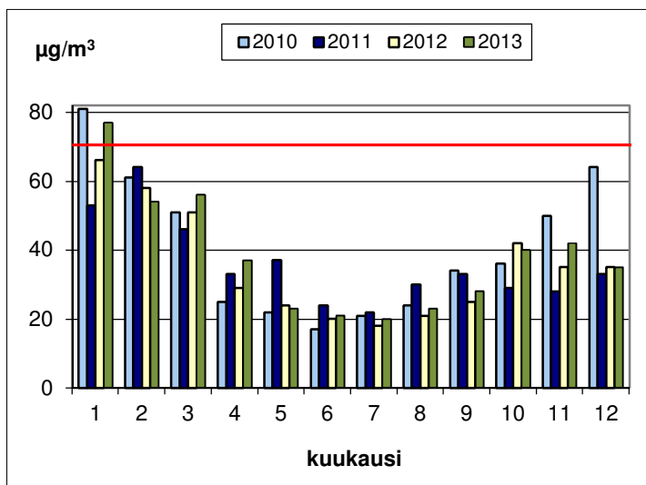
Kuva 34. Typpidioksidipitoisuuden ohjearvoon verrattavat vuorokausikeskiarvot Raisiossa vuosina 2010 – 2013.
