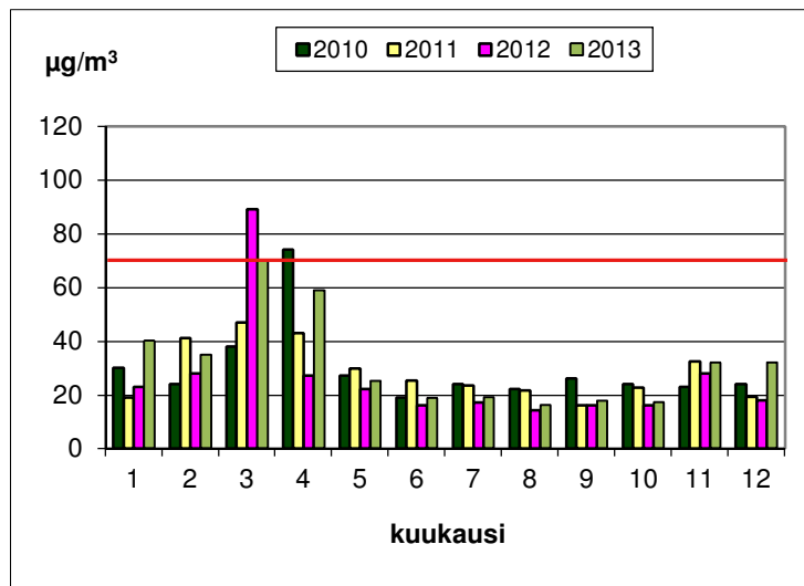
Kuva 19. Hengitettävien hiukkasten ohjearvoon ( 70 \mu\text{g}/\text{m}^3 ) verrattavat vuorokausikeskiarvot Kauppatorilla vuosina 2010 - 2013. Joulukuussa 2013 tulosten saatavuusprosentti oli vain 80.
