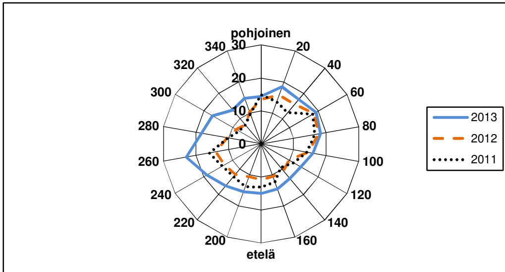
Kuva 18. Orikedon typpidioksidin keskipitoisuus ( \mu\text{g}/\text{m}^3 ) eri tuulensuunnilla vuosina 2011, 2012 ja 2013.
