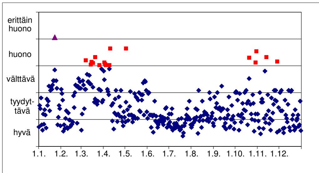
Kuva 29. Raision ilmanlaatu indeksillä kuvattuna vuonna 2013.
