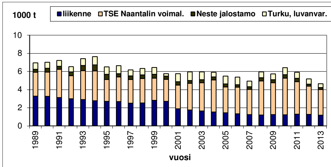
Kuva 2. Ympäristönsuojelulain nojalla luvanvaraisten laitosten sekä liikenteen typpioksidipäästöjen kehitys Turun seudulla.
