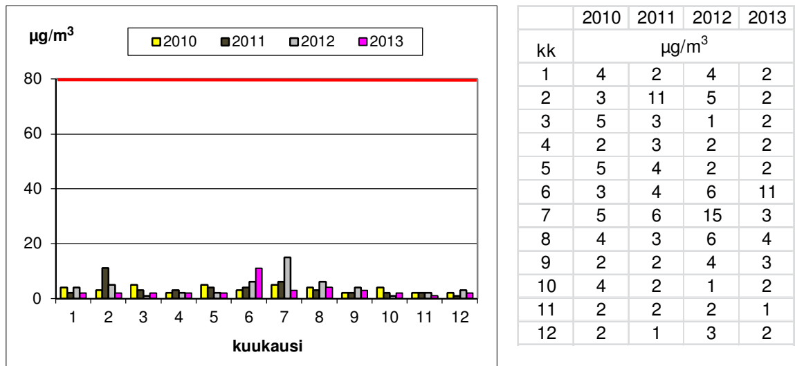
Kuva 31. Kaanaan vuorokausiohjearvoon (80 µg/m 3 ) verrattavat rikkidioksidipitoisuudet vuosina 2010 - 2013.
