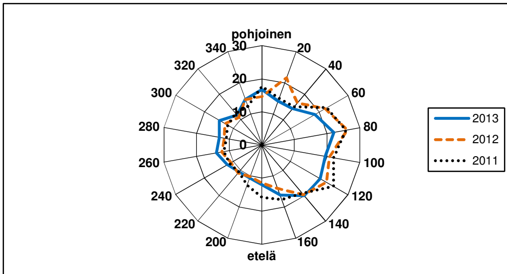
Kuva 48. Naantalin typpidioksidin keskipitoisuus ( \mu\text{g}/\text{m}^3 ) eri tuulen suunnilla vuosina 2011, 2012 ja 2013.
