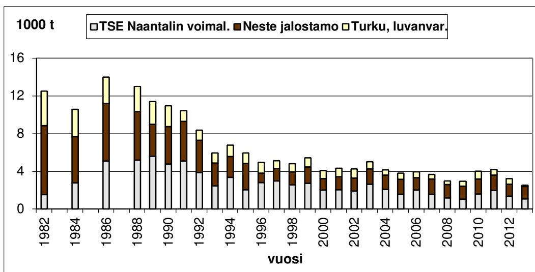
Kuva 1. Ympäristönsuojelulain nojalla luvanvaraisten laitosten rikkidioksidipäästöjen kehitys Turun seudulla.
