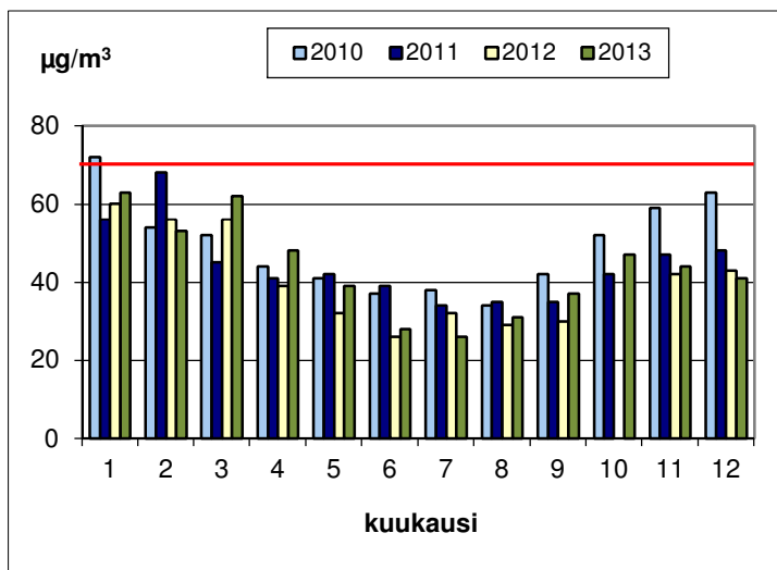
Kuva 13. Typpidioksidipitoisuuden ohjearvoon verrattavat vuorokausikeskiarvot Turun Kauppatorilla vuosina 2010 – 2013. Kesäkuussa 2010 mittausten ajallinen kattavuus oli vain 71 % ja lokakuussa 2012 81 %.
