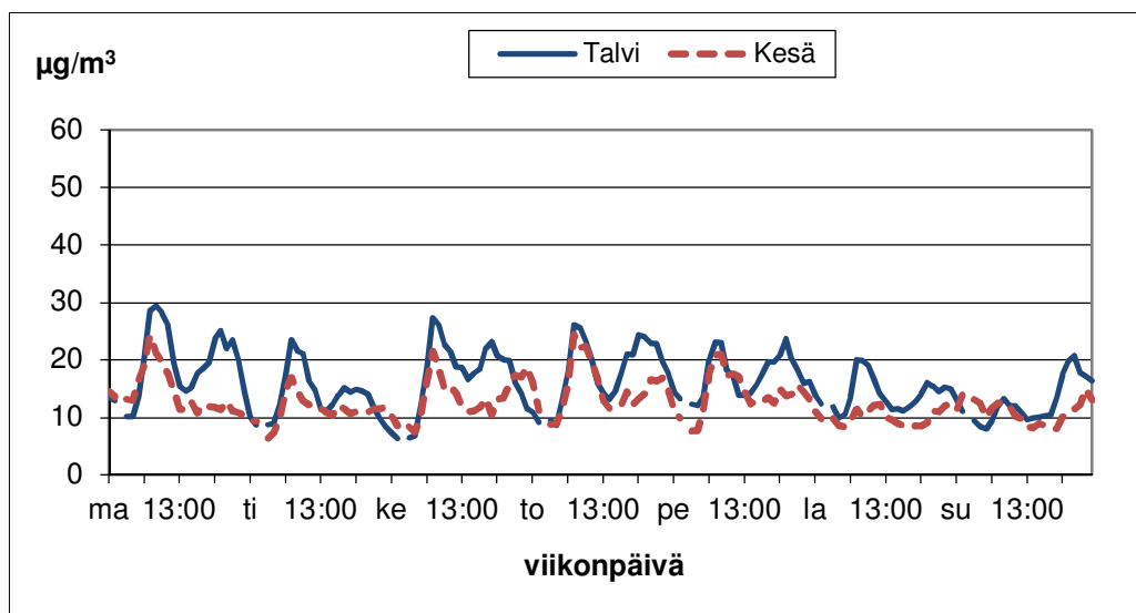
Kuva 47. Naantalissa typpidioksidipitoisuuden vaihtelut viikon eri ajankohtina kesällä (1.4.–30.9.) ja talvella (1.1.–31.3. ja 1.10.–31.12.) vuonna 2013.
