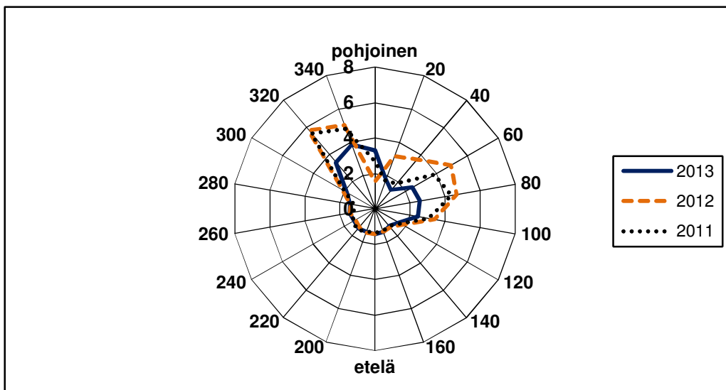
Kuva 11. Ruissalon rikkidioksidin keskipitoisuus ( \mu\text{g}/\text{m}^3 ) eri tuulen suunnilla vuosina 2011, 2012 ja 2013.
