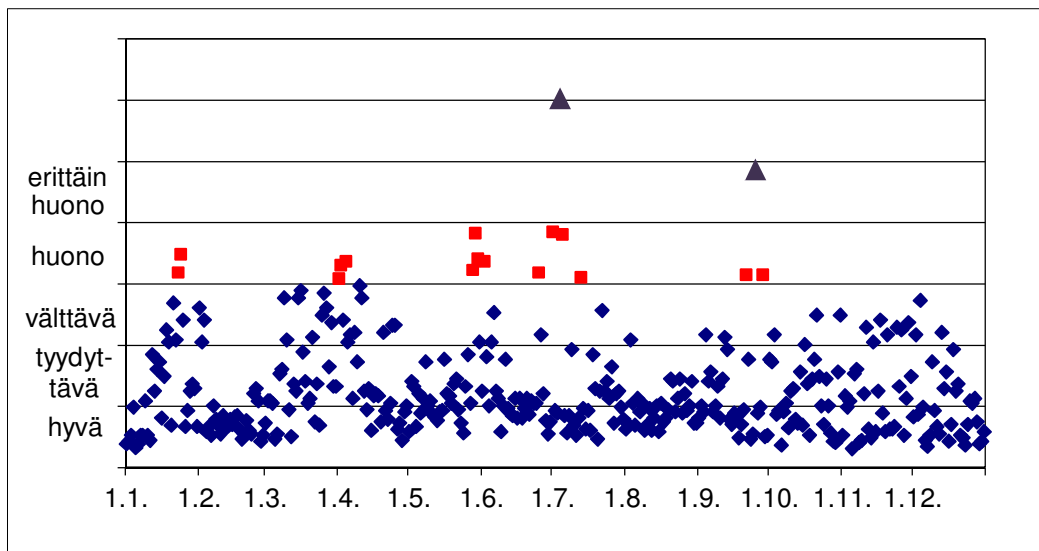
Kuva 51. Kaarinan ilmanlaatu indeksillä kuvattuna vuonna 2013.
