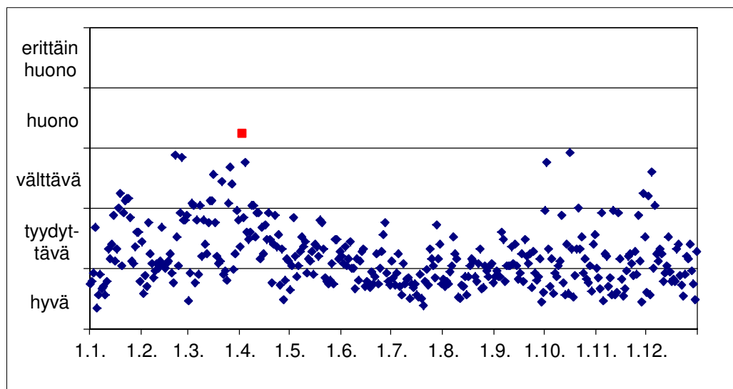
Kuva 8. Turun Orikedon ilmanlaatu indeksillä kuvattuna vuonna 2013.
