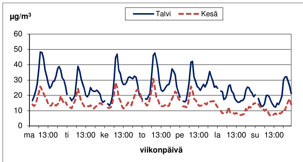
Kuva 36. Raision typpidioksidipitoisuuden vaihtelut viikon eri ajankohtina kesällä (1.4.–30.9.) ja talvella (1.1.–31.3. ja 1.10.–31.12.) vuonna 2013.
