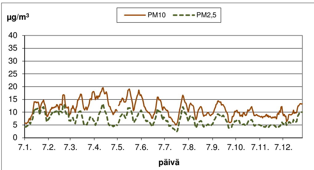
Kuva 23. Orikedon hengitettävien ja pienhiukkasten vuorokausiarvojen seitsemän päivän liukuvat keskiarvot vuonna 2013.
