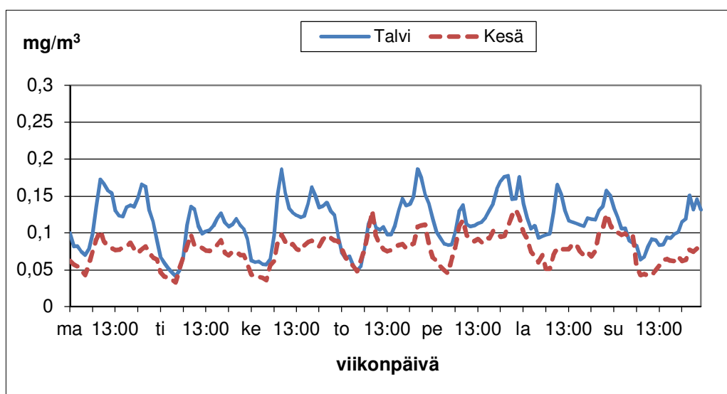
Kuva 25. Kauppatorin hiilimonoksidin pitoisuuden vaihtelut viikon eri ajankohtina kesällä (1.4.-30.9.) ja talvella (1.1.-31.3. ja 1.10.-31.12.) vuonna 2013.
