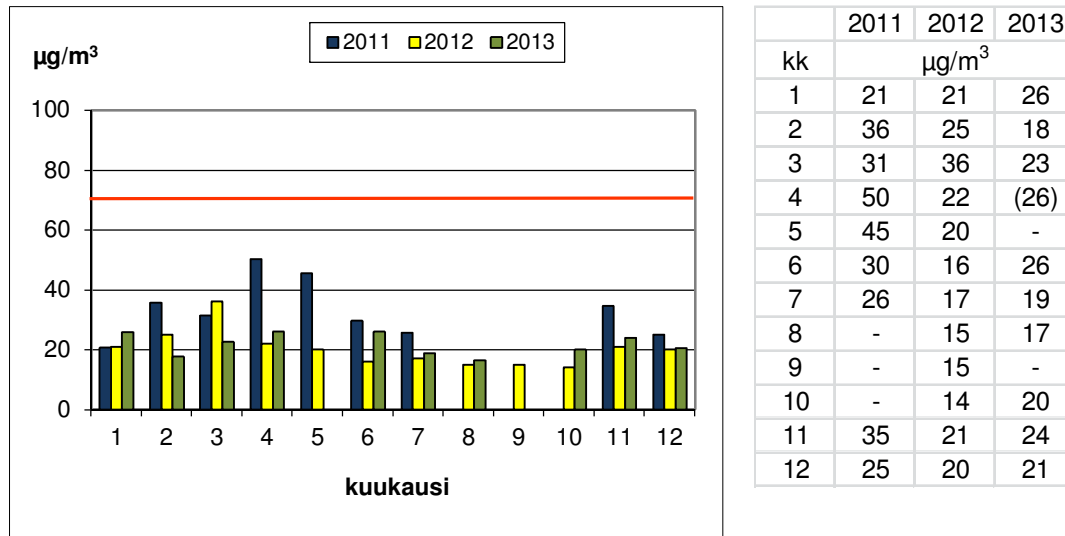
Kuva 59. Hengitettävien hiukkasten ohjearvoon (70 µg/m 3 ) verrattavat vuorokausikeskiarvot Paraisilla vuosina 2011, 2012 ja 2013. Laitteivian vuoksi elo-, syys- ja lokakuun 2011 sekä touko- ja syyskuun 2013 mittaustulokset puuttuvat. Huhtikuun 2013 tulosten saatavuusprosentti oli 50. Mittauspaikkaa on vaihdettu vuosittain.
