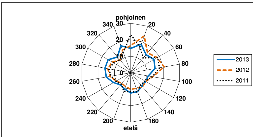
Kuva 55. Kaarinan typpidioksidin keskipitoisuus ( \mu\text{g}/\text{m}^3 ) eri tuulen suunnilla vuosina 2011, 2012 ja 2013.
