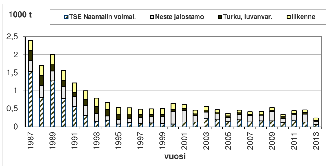
Kuva 3. Ympäristönsuojelulain nojalla luvanvaraisten laitosten sekä liikenteen hiukkaspäästöjen kehitys Turun seudulla.
