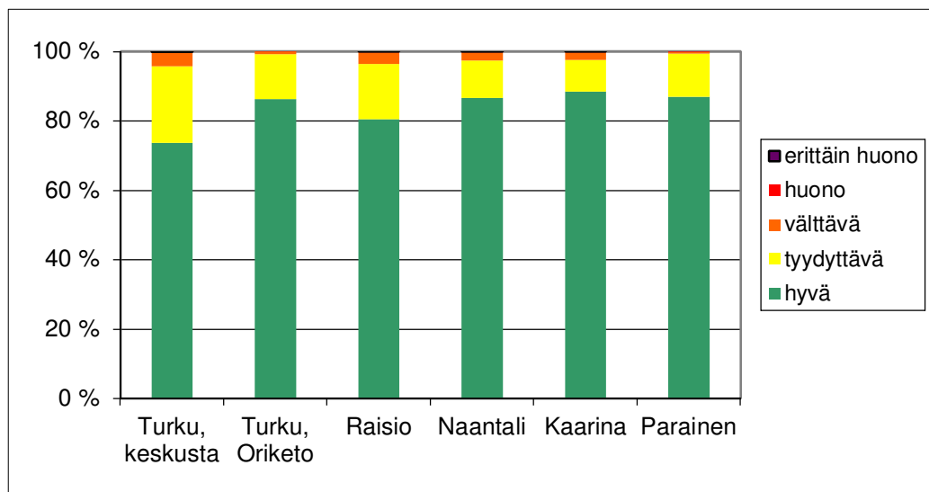
Kuva 6. Ilmanlaatuindeksin jakautuminen tunneittain eri luokkiin vuonna 2013.
