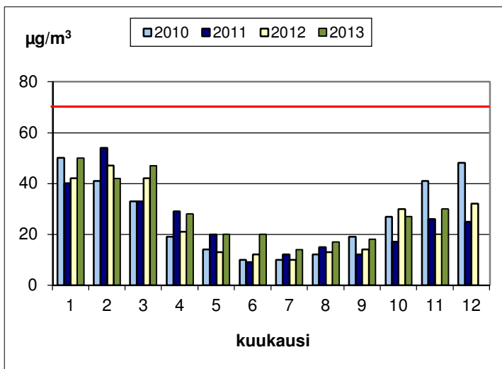
Kuva 15. Typpidioksidipitoisuuden ohjearvoon verrattavat vuorokausikeskiarvot Turun Orikedolla vuosina 2010 - 2013. Toukokuussa 2010 mittausten ajallinen kattavuus oli vain 81 %, kesäkuussa 2012 77 % ja heinäkuussa 87 %. Joulukuun 2013 ohjearvovertailu puuttuu laitteen vuoksi.
