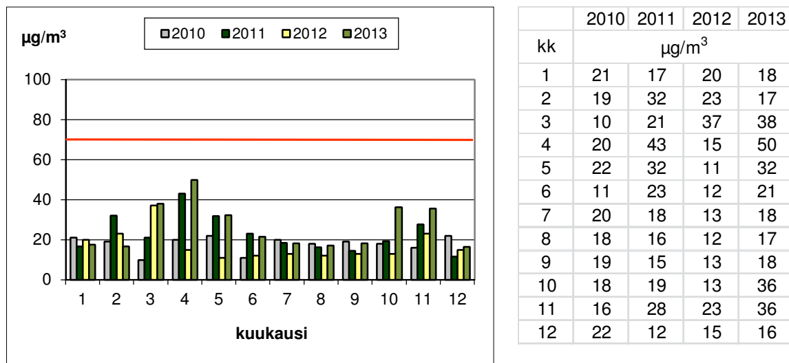
Kuva 38. Hengitettävien hiukkasten ohjearvoon ( 70 \mu\text{g}/\text{m}^3 ) verrattavat vuorokausikeskiarvot Raisiossa vuosina 2010 - 2013.
