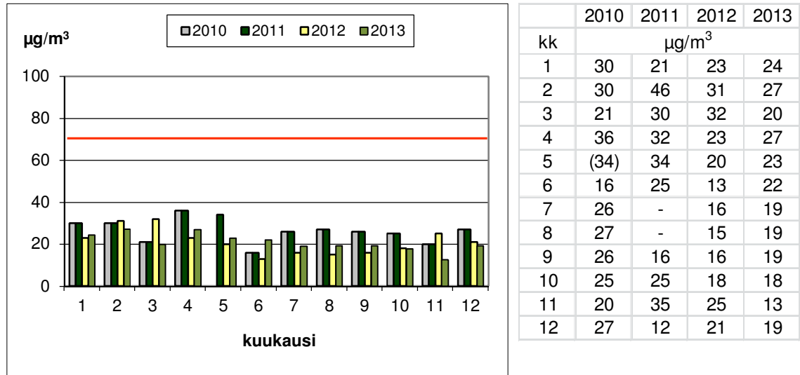
Kuva 20. Hengitettävien hiukkasten ohjearvoon ( 70 \mu\text{g}/\text{m}^3 ) verrattavat vuorokausikeskiarvot Oriekedolla vuosina 2010 – 2013. Toukokuussa 2010 mittausten ajallinen kattavuus oli vain 82 %. Heinä- ja elokuu 2011 puuttuvat laitevian vuoksi.
