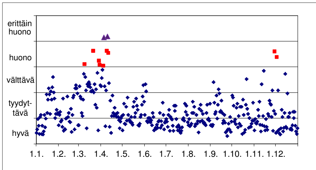
Kuva 40. Naantalin keskustan ilmanlaatu indeksillä kuvattuna vuonna 2013.
