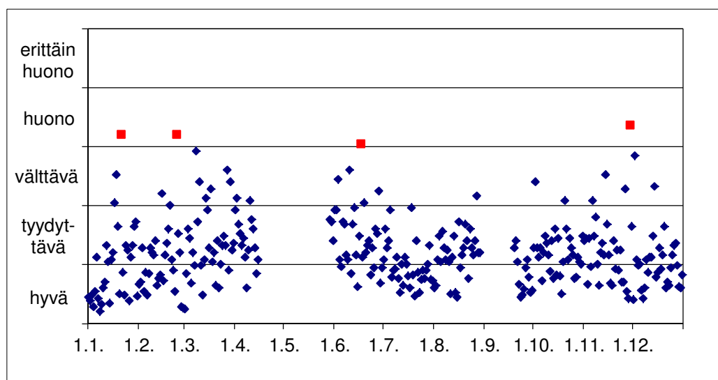
Kuva 58. Paraisten ilmanlaatu indeksillä kuvattuna vuonna 2013.
