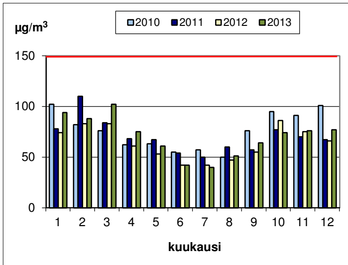
Kuva 14. Typpidioksidin ohjearvoon verrattavat tuntikeskiarvot Turun Kauppatorilla vuosina 2010 - 2013. Kesäkuussa 2010 mittausten ajallinen kattavuus oli 71 % ja lokakuussa 2012 81 %.
