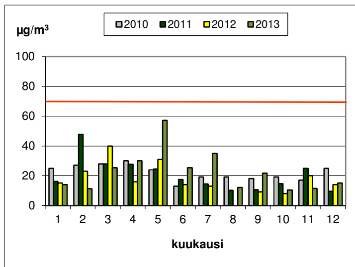
Kuva 56. Hengitettävien hiukkasten ohjearvoon ( 70 \mu\text{g}/\text{m}^3 ) verrattavat vuorokausikeskiarvot Kaarinassa vuosina 2010 - 2013. Elokuulta 2012 ei ole mittaustuloksia laitevian vuoksi.
