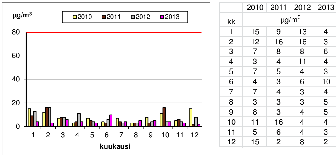
Kuva 10. Ruissalon vuorokausiohjearvoon verrattavat rikkidioksidipitoisuudet vuosina 2010 - 2013. Vuorokausiohjearvo on 80 \mu\text{g}/\text{m}^3 .
