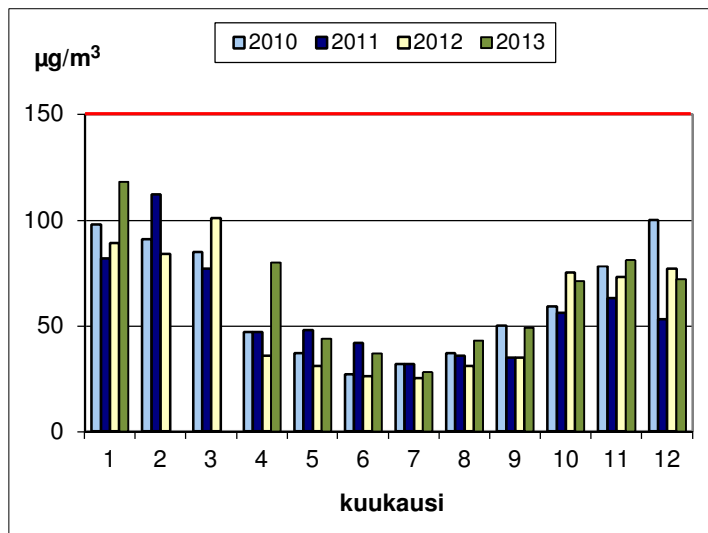
Kuva 53. Typpidioksidin ohjearvoon verrattavat tuntikeskiarvot Kaarinassa vuosina 2010 – 2013. Huhtikuussa 2010 tulosten ajallinen kattavuus oli vain 78 %, tammikuussa 2012 86 % ja syyskuussa 2012 84 %. Helmi- ja maaliskuun 2013 tulokset puuttuvat laitevian vuoksi.
