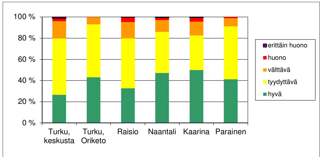
Kuva 5. Ilmanlaatuindeksin päivittäisten maksimiarvojen jakautuminen eri luokkiin vuonna 2013.
