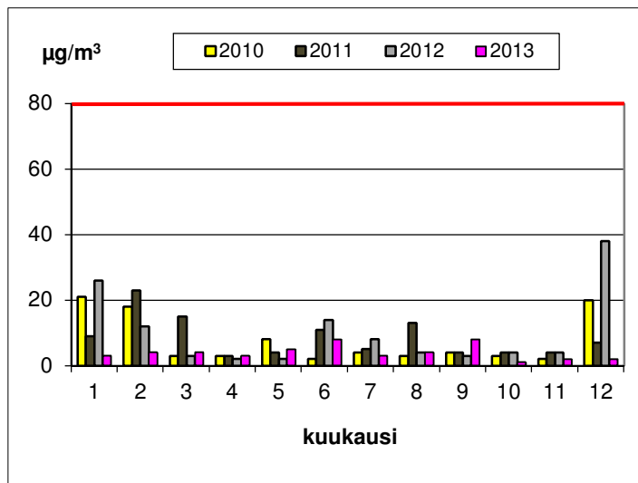
Kuva 42. Vuorokausiohjearvoon (80 µg/m 3 ) verrattavat rikkidioksidipitoisuudet Naantalissa vuosina 2010 - 2013.
