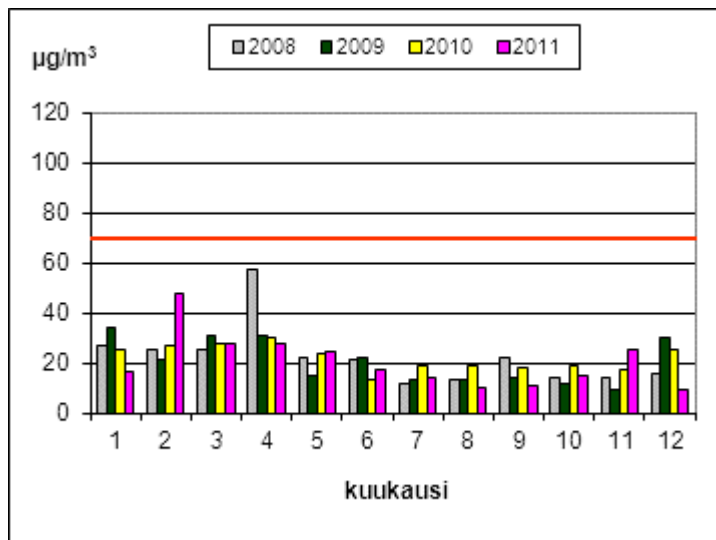
Kuva 56. Hengitettävien hiukkasten ohjearvoon ( 70 \mu\text{g}/\text{m}^3 ) verrattavat vuorokausikeskiarvot Kaarinassa vuosina 2008 - 2011.
