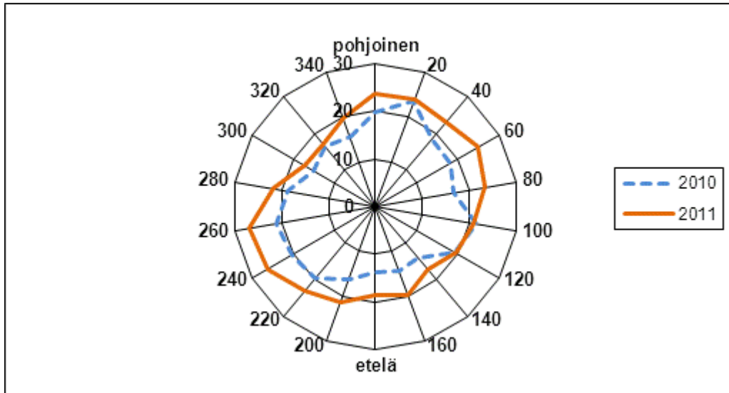
Kuva 37. Raision typpidioksidin keskipitoisuus ( \mu\text{g}/\text{m}^3 ) eri tuulen suunnilla vuosina 2010 ja 2011.
