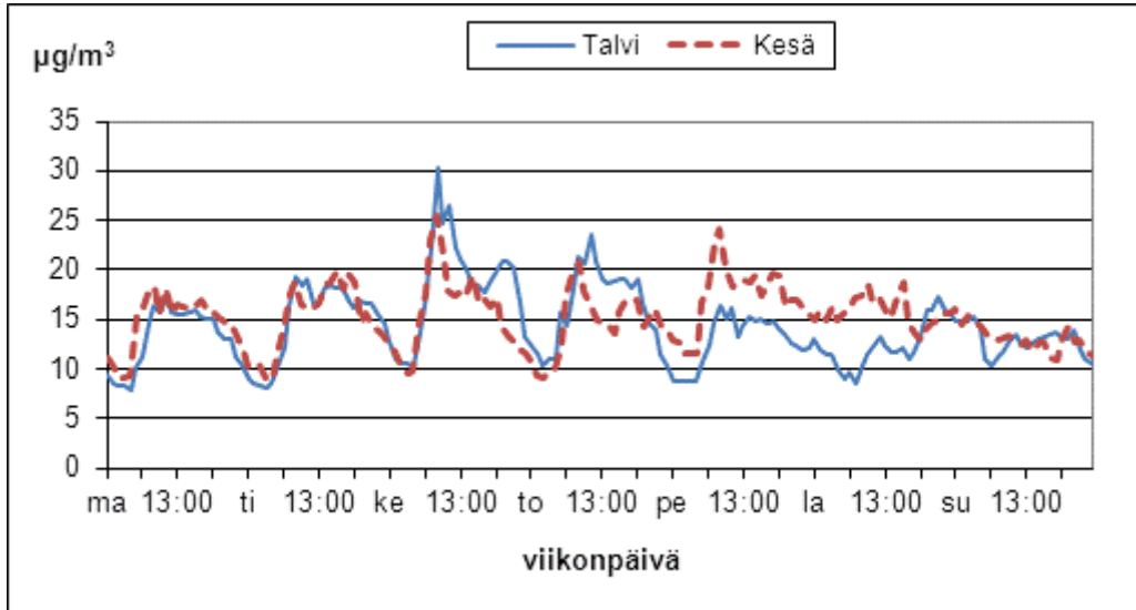
Kuva 22. Kauppatorin hengitettävien hiukkasten pitoisuuden vaihtelut viikon eri ajankohtina kesällä (1.4.–30.9.) ja talvella (1.1.–31.3. ja 1.10.–31.12.) vuonna 2011.
