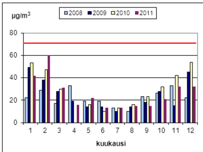
Kuva 52. Typpidioksidipitoisuuden ohjearvoon verrattavat vuorokausikeskiarvot Kaarinassa vuosina 2008 - 2011. Huhtikuussa 2010 tulosten ajallinen kattavuus oli vain 78 %.
