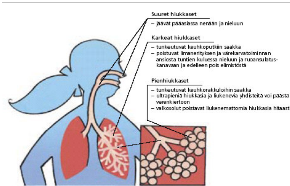
Kuva 62. Hiukkasten pääsy elimistöön (Hengitysliitto, 2004).
