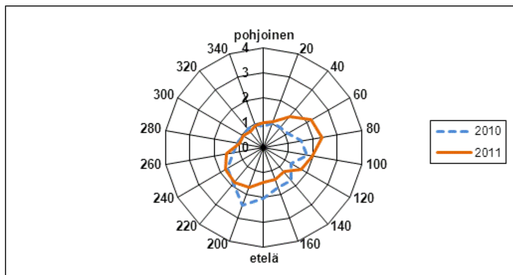
Kuva 32. Kaanaan rikkidioksidin keskipitoisuus ( \mu\text{g}/\text{m}^3 ) eri tuulen suunnilla vuosina 2010 ja 2011.
