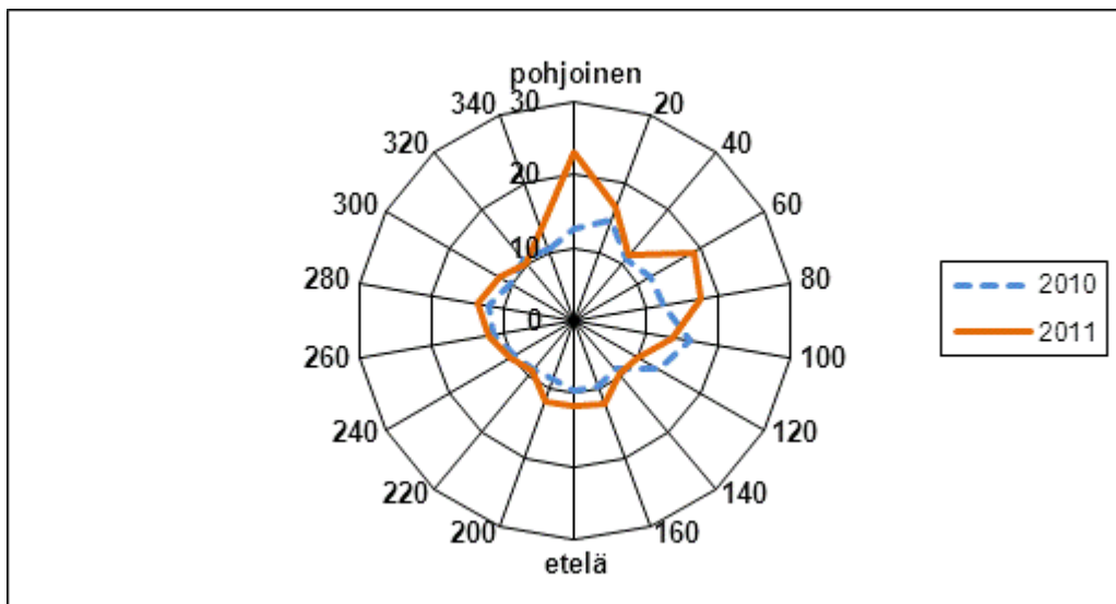
Kuva 55. Kaarinan typpidioksidin keskipitoisuus ( \mu\text{g}/\text{m}^3 ) eri tuulen suunnilla vuosina 2010 ja 2011.
