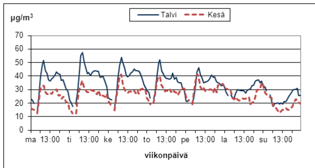
Kuva 17. Kauppatorin typpidioksidipitoisuuden vaihtelut viikon eri ajankohtina kesällä (1.4.–30.9.) ja talvella (1.1.–31.3. ja 1.10.–31.12.) vuonna 2011.
