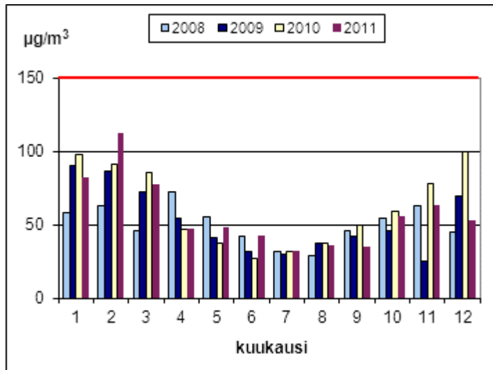
Kuva 53. Typpidioksidin ohjearvoon verrattavat tuntikeskiarvot Kaarinassa vuosina 2008 – 2011. Huhtikuussa 2010 tulosten ajallinen kattavuus oli vain 78 %.
