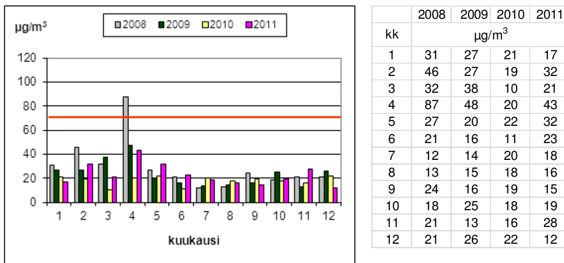
Kuva 38. Hengitettävien hiukkasten ohjearvoon ( 70 \mu\text{g}/\text{m}^3 ) verrattavat vuorokausikeskiarvot Raisiossa vuosina 2008 - 2011.
