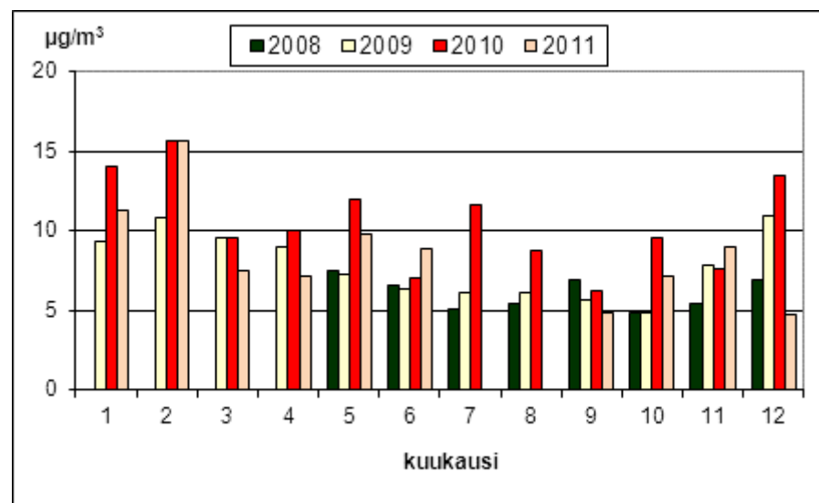
Kuva 21. Orikedon pienhiukkaspitoisuuden ( PM_{2,5} ) kuukausikeskiarvot vuosina 2008 - 2011. Heinä- ja elokuu 2011 puuttuvat laitevian vuoksi.
