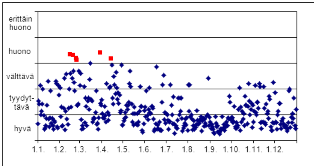
Kuva 51. Kaarinan ilmanlaatu indeksillä kuvattuna vuonna 2011.
