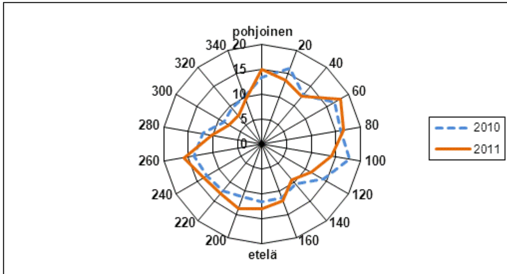
Kuva 18. Orikedon typpidioksidin keskipitoisuus ( \mu\text{g}/\text{m}^3 ) eri tuulensuunnilla vuosina 2010 ja 2011.
