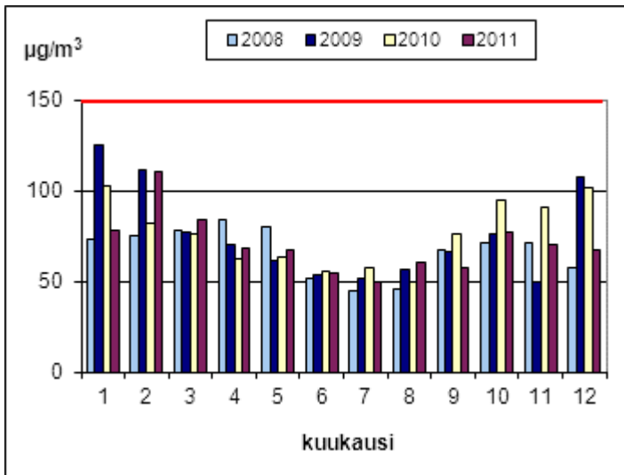
Kuva 14. Typpidioksidin ohjearvoon verrattavat tuntikeskiarvot Turun Kauppatorilla vuosina 2008 - 2011. Kesäkuussa 2010 mittausten ajallinen kattavuus oli 71 %.
