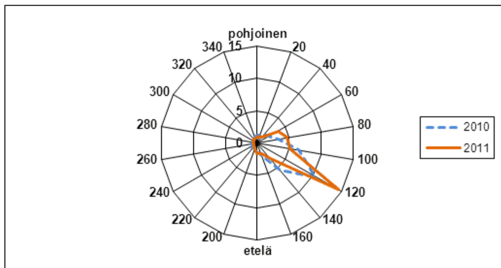
Kuva 43. Naantalin rikkidioksidin keskipitoisuus (µg/m 3 ) eri tuulen suunnilla vuosina 2010 ja 2011.
