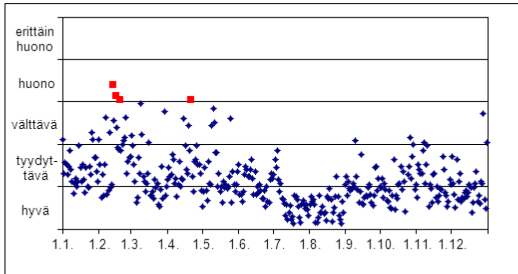
Kuva 8. Turun Orikedon ilmanlaatu indeksillä kuvattuna vuonna 2011.
