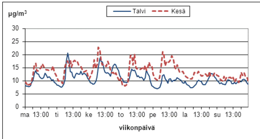
Kuva 39. Raision hengitettävien hiukkasten pitoisuuden vaihtelut viikon eri ajankohtina kesällä (1.4.–30.9.) ja talvella (1.1.–31.3. ja 1.10.–31.12.) vuonna 2011.
