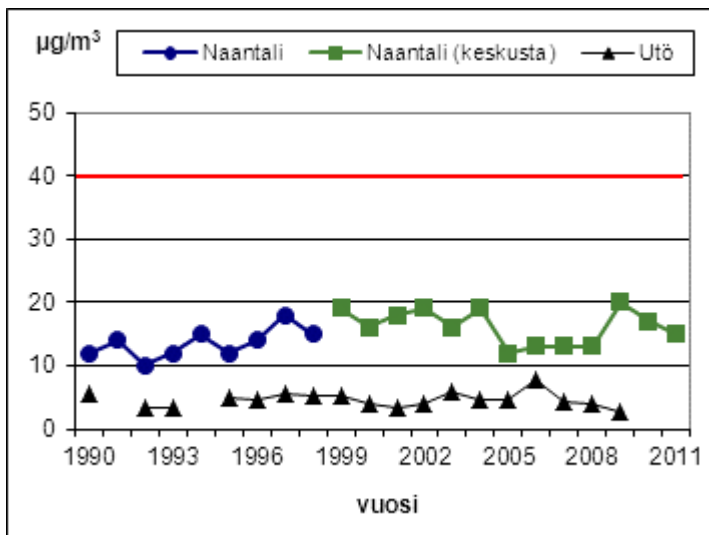
Kuva 44. Typpidioksidipitoisuuden vuosikeskiarvot Naantalissa ja Utössä.
