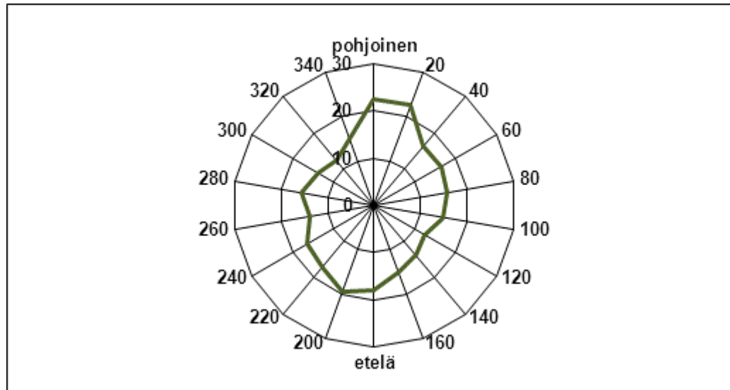
Kuva 61. Paraisten hengitettävien hiukkasten keskipitoisuus ( \mu\text{g}/\text{m}^3 ) eri tuulen suunnilla vuonna 2011.
