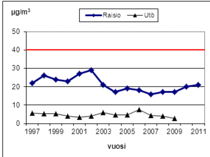
Kuva 33. Typidioksidipitoisuuden vuosikeskiarvot Raisiossa ja Utössä. Raision mittauspisteen paikkaa on siirretty elokuussa 2002.
