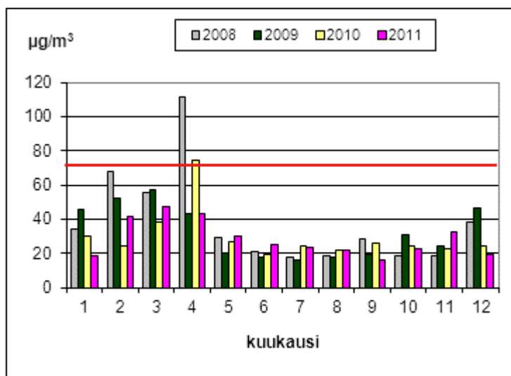
Kuva 19. Hengitettävien hiukkasten ohjearvoon ( 70 \mu\text{g}/\text{m}^3 ) verrattavat vuorokausikeskiarvot Kauppatorilla vuosina 2008 - 2011.
