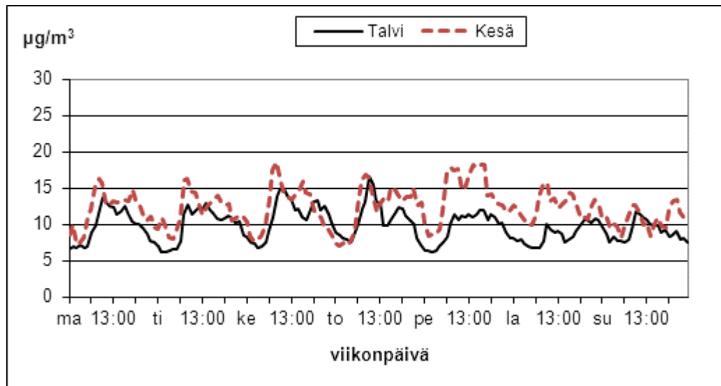
Kuva 50. Naantalin hengitettävien hiukkasten pitoisuuksien vaihtelut viikon eri ajankohtina kesällä (1.4.–30.9.) ja talvella (1.1.–31.3. ja 1.10.–31.12.) vuonna 2011.
