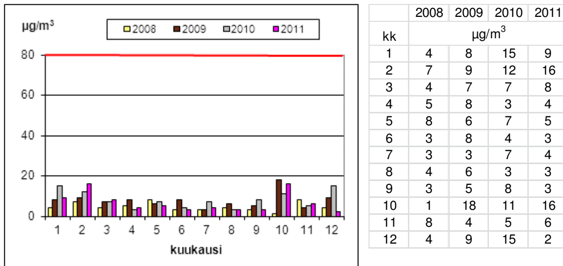
Kuva 10. Ruissalon vuorokausiohjearvoon verrattavat rikkidioksidipitoisuudet vuosina 2008 - 2011. Vuorokausiohjearvo on 80 µg/m 3 .
