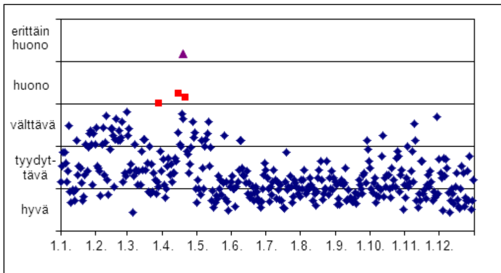
Kuva 29. Raision ilmanlaatu indeksillä kuvattuna vuonna 2011.
