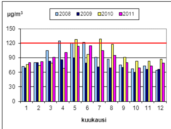
Kuva 26. Otsonipitoisuuksien korkeimmat 8 tunnin keskiarvot Ruissalossa vuosina 2008 – 2011. Huhtikuussa 2010 mittausten ajallinen kattavuus oli vain 35 %.
