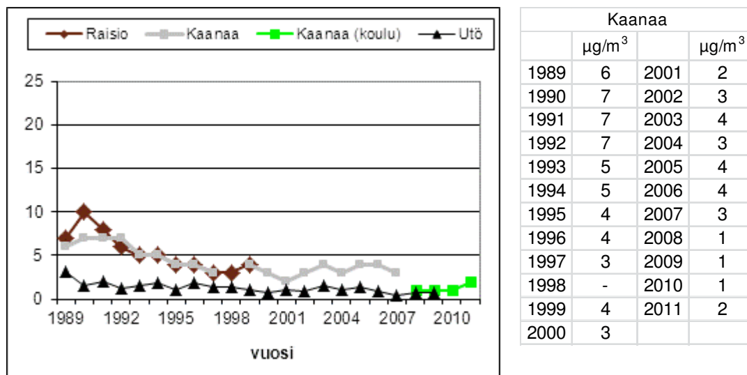
Kuva 30. Rikkidioksidipitoisuuden vuosikeskiarvojen kehitys Raision keskustassa, Kaanaalla ja Utössä.
