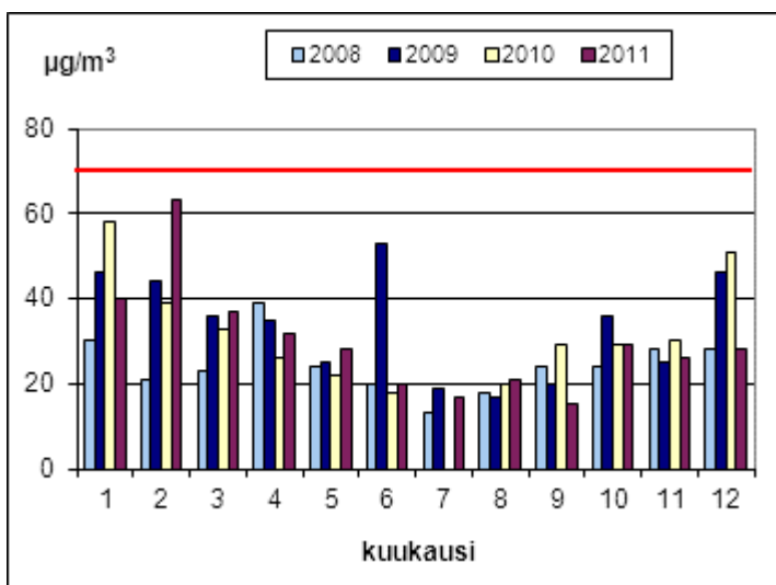
Kuva 45. Typpidioksidipitoisuuden ohjearvoon verrattavat vuorokausikeskiarvot Naantalissa vuosina 2008 – 2011. Heinäkuussa 2010 mittausten ajallinen kattavuus oli vain 85 %.
