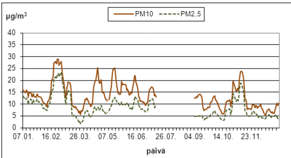
Kuva 23. Orikedon hengitettävien ja pienhiukkasten vuorokausiarvojen seitsemän päivän liukuvat keskiarvot vuonna 2011.
