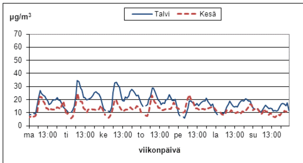
Kuva 47. Naantalien typpidioksidipitoisuuden vaihtelut viikon eri ajankohtina kesällä (1.4.–30.9.) ja talvella (1.1.–31.3. ja 1.10.–31.12.) vuonna 2011.
