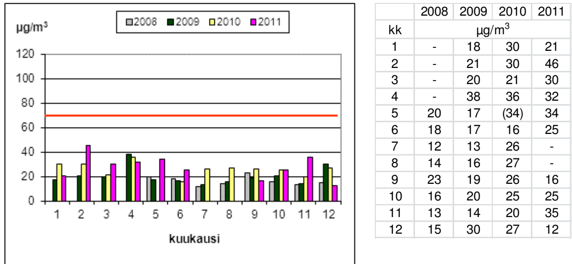
Kuva 20. Hengitettävien hiukkasten ohjearvoon ( 70 \mu\text{g}/\text{m}^3 ) verrattavat vuorokausikeskiarvot Orikedolla vuosina 2008 – 2011. Toukokuussa 2010 mittausausten ajallinen kattavuus oli vain 82 %. Heinä- ja elokuu 2011 puuttuvat laitevian vuoksi.
