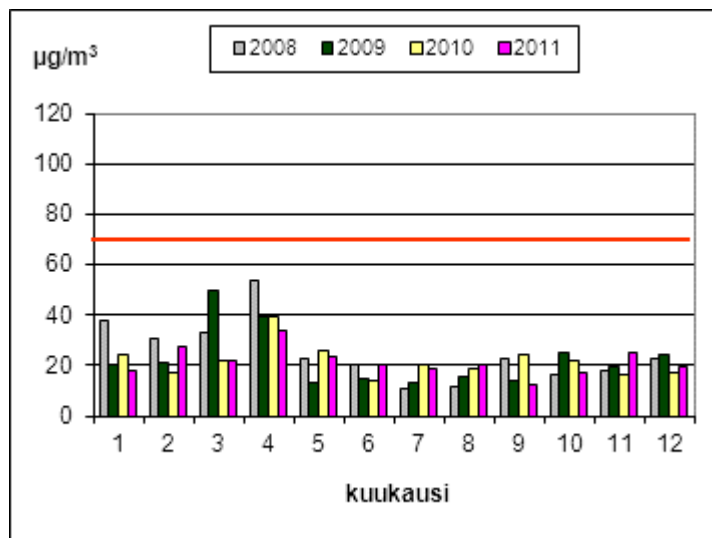
Kuva 49. Hengitettävien hiukkasten ohjearvoon ( 70 \mu\text{g}/\text{m}^3 ) verrattavat vuorokausikeskiarvot Naantalissa vuosina 2008 - 2011.
