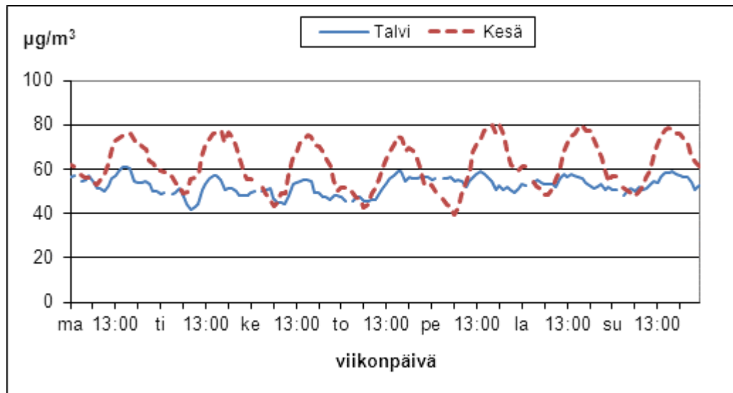
Kuva 28. Ruissalon otsonipitoisuuden vaihtelut viikon eri ajankohtina kesällä (1.4.–30.9.) ja talvella (1.1.–31.3. ja 1.10.–31.12.) vuonna 2011.
