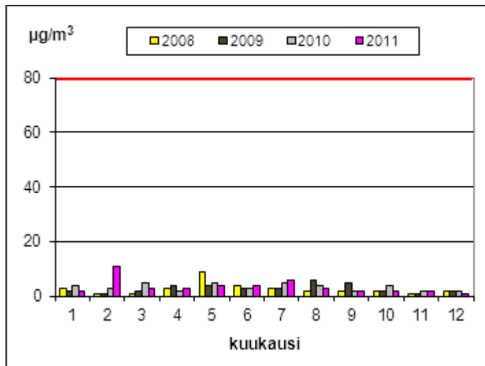
Kuva 31. Kaanaan vuorokausi-ohjearvoon ( 80 \mu\text{g}/\text{m}^3 ) verrattavat rikkidioksidipitoisuudet vuosina 2008 - 2011. Tammikuussa 2008 tulosten ajallinen kattavuus oli vain 65 %.
