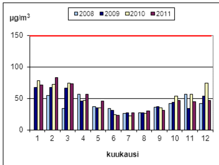
Kuva 16. Typpidioksidipitoisuuden ohjearvoon verrattavat tuntikeskiarvot Turun Orikedolla vuosina 2008 – 2011. Toukokuussa 2010 mittausten ajallinen kattavuus oli vain 81 %.
