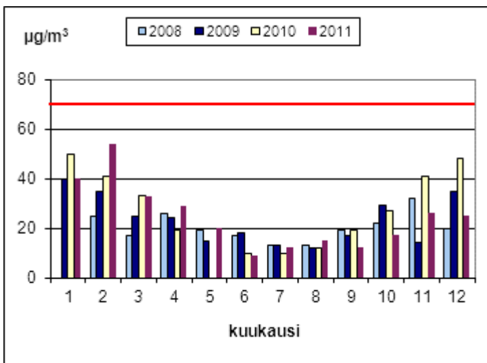
Kuva 15. Typpidioksidipitoisuuden ohjearvoon verrattavat vuorokausikeskiarvot Turun Orikedolla vuosina 2008 – 2011. Toukokuussa 2010 mittausten ajallinen kattavuus oli vain 81 %.
