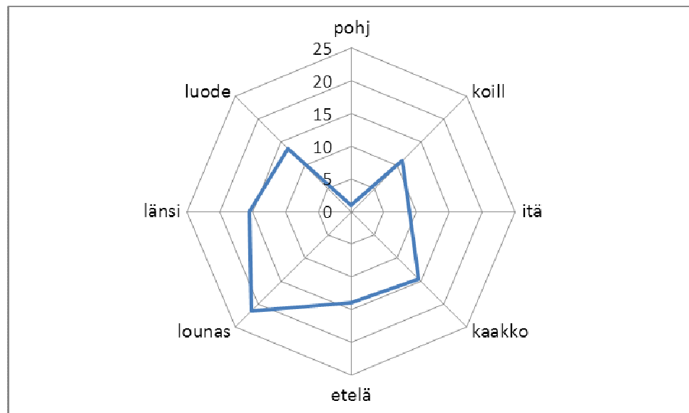
Kuva 4. Tuulensuunnan jakautuminen Turun Juhannuskukkulalla vuonna 2011.
