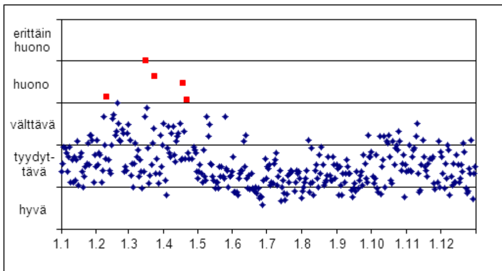
Kuva 7. Turun keskustan ilmanlaatu indeksillä kuvattuna vuonna 2011.
