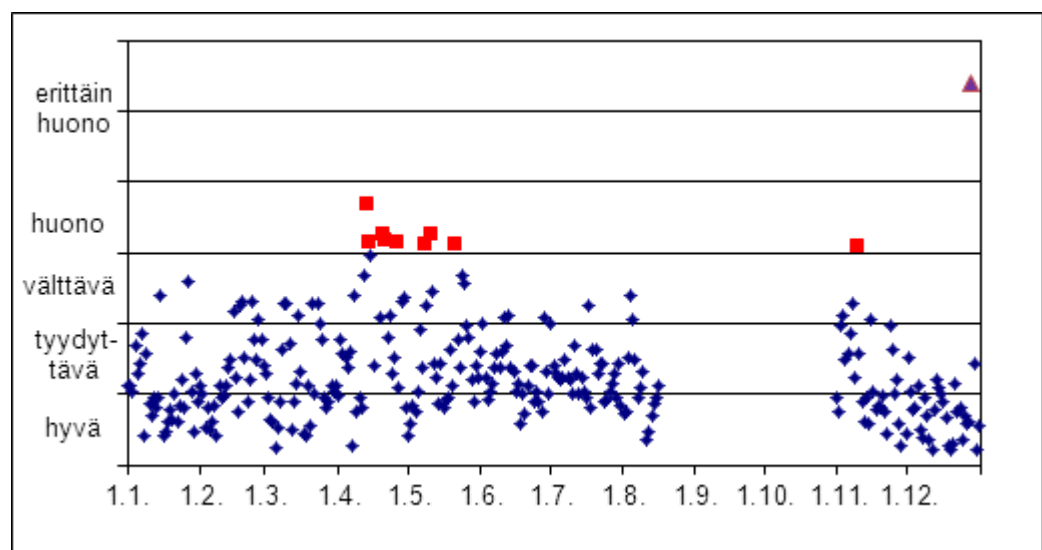
Kuva 58. Paraisten ilmanlaatu indeksillä kuvattuna vuonna 2011.
