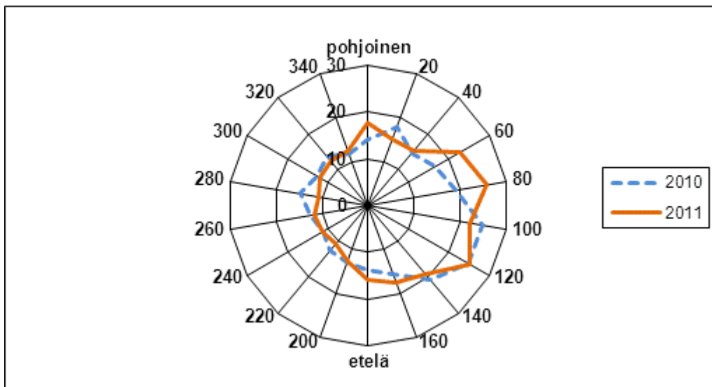
Kuva 48. Naantalin typpidioksidin keskipitoisuus ( \mu\text{g}/\text{m}^3 ) eri tuulen suunnilla vuosina 2010 ja 2011.
