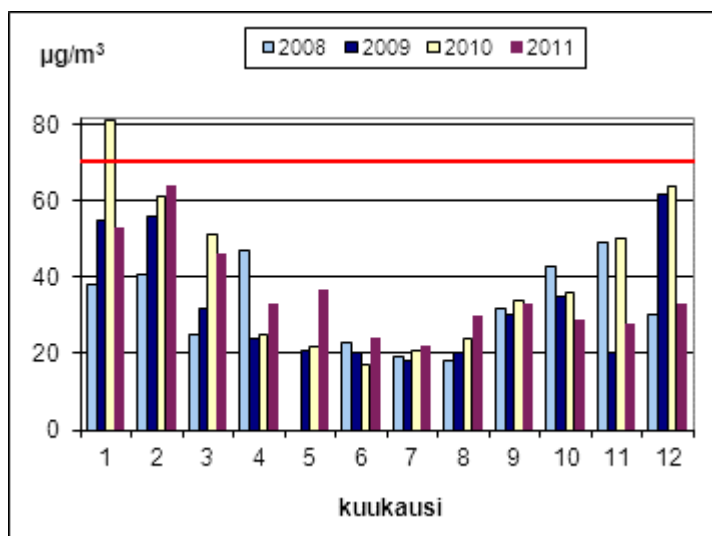
Kuva 34. Typidioksidipitoisuuden ohjearvoon verrattavat vuorokausikeskiarvot Raisiossa vuosina 2008 – 2011. Huhti- ja kesäkuun 2008 mittausten ajalliset kattavuudet olivat vain 65 ja 60 %. Toukokuulta 2008 ei ole mittaus tuloksia.
