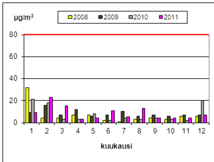
Kuva 42. Vuorokausiohjearvoon (80 µg/m 3 ) verrattavat rikkidioksidipitoisuudet Naantalissa vuosina 2008 - 2011.
