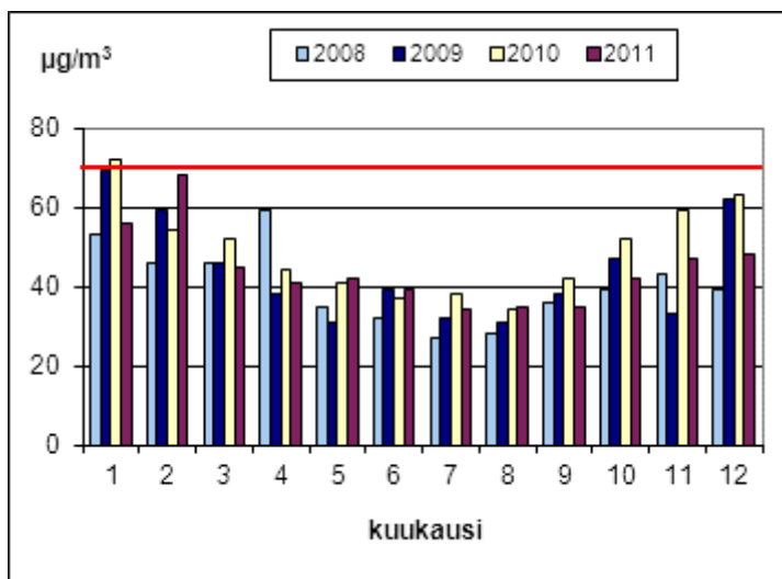
Kuva 13. Typpidioksidipitoisuuden ohjearvoon verrattavat vuorokausikeskiarvot Turun Kauppatorilla vuosina 2008 – 2011. Kesäkuussa 2010 mittauksen ajallinen kattavuus oli vain 71 %.
