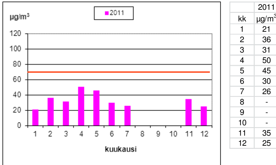
Kuva 59. Hengitettävien hiukkasten ohjearvoon (70 µg/m 3 ) verrattavat vuorokausikeskiarvot Paraisilla vuonna 2011. Laitevian vuoksi elo-, syys- ja loka-kuun mittaustulokset puuttuvat.
