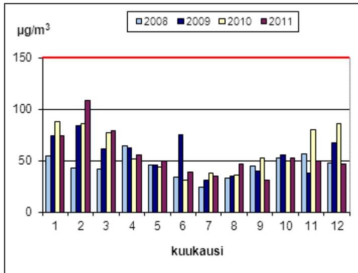
Kuva 46. Typpidioksidin ohjearvoon verrattavat tuntikeskiarvot Naantalissa vuosina 2008 - 2011. Heinäkuussa 2010 mittausten ajallinen kattavuus oli vain 85 %.
