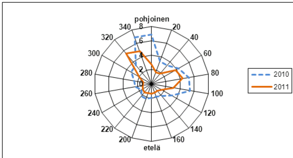
Kuva 11. Ruissalon rikkidioksidin keskipitoisuus (µg/m 3 ) eri tuulen suunnilla vuosina 2010 ja 2011.
