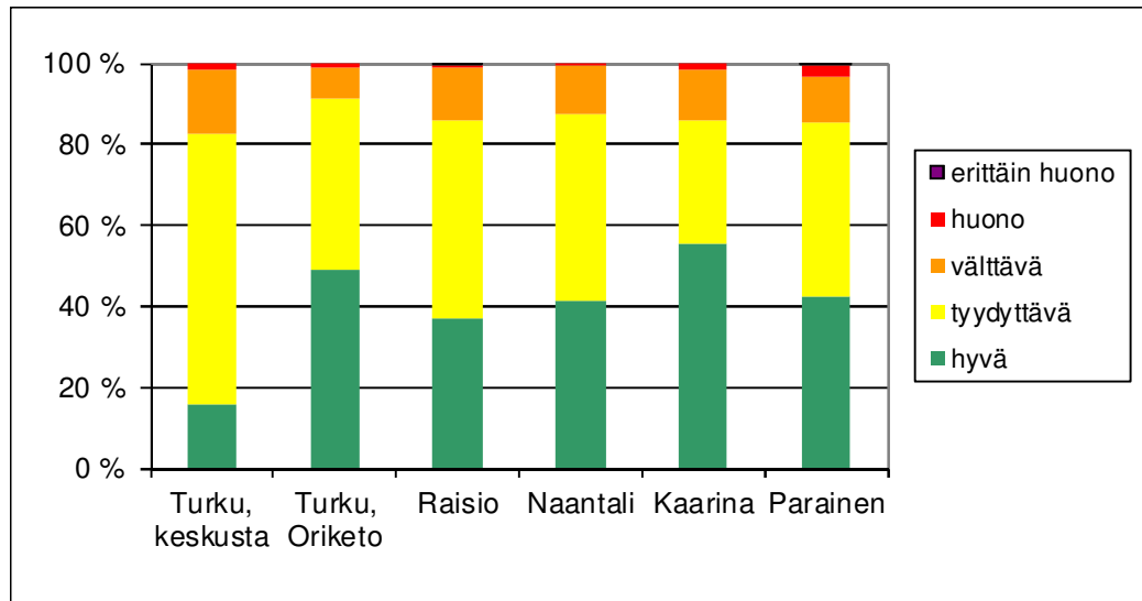
Kuva 5. Ilmanlaatuindeksin päivittäisten maksimiarvojen jakautuminen eri luokkiin vuonna 2011.
