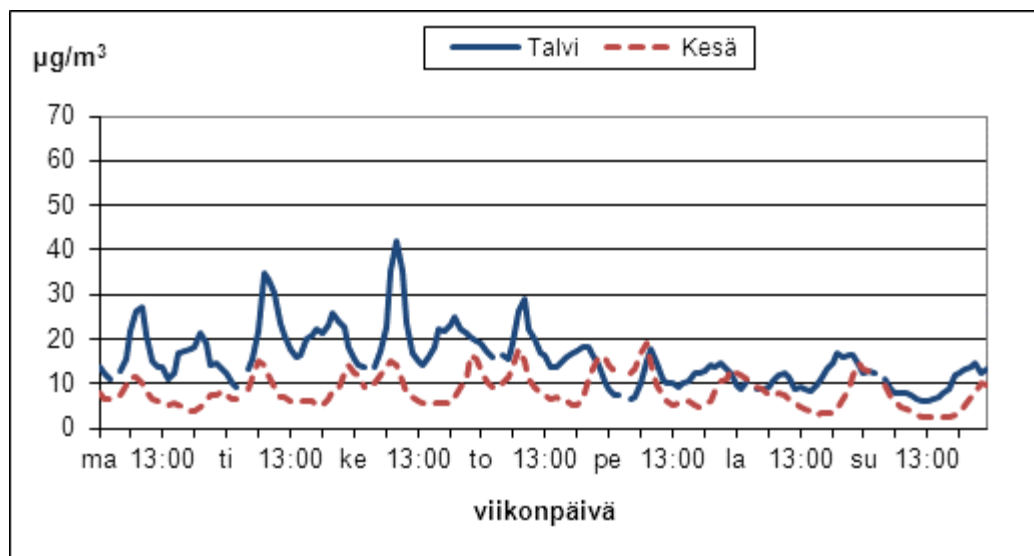
Kuva 54. Kaarinan typpidioksidipitoisuuden vaihtelut viikon eri ajankohtina kesällä (1.4.–30.9.) ja talvella (1.1.–31.3. ja 1.10.–31.12.) vuonna 2011.
