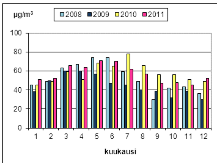
Kuva 27. Otsonipitoisuuksien kuukausikeskiarvot Ruissalossa vuosina 2008 - 2011.
