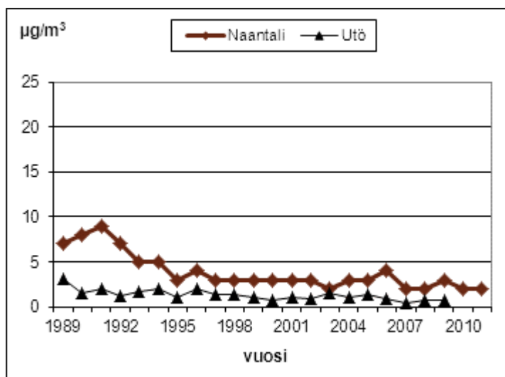
Kuva 41. Rikkidioksidipitoisuuden vuosikeskiarvojen kehitys Naantalissa ja Utössä.
