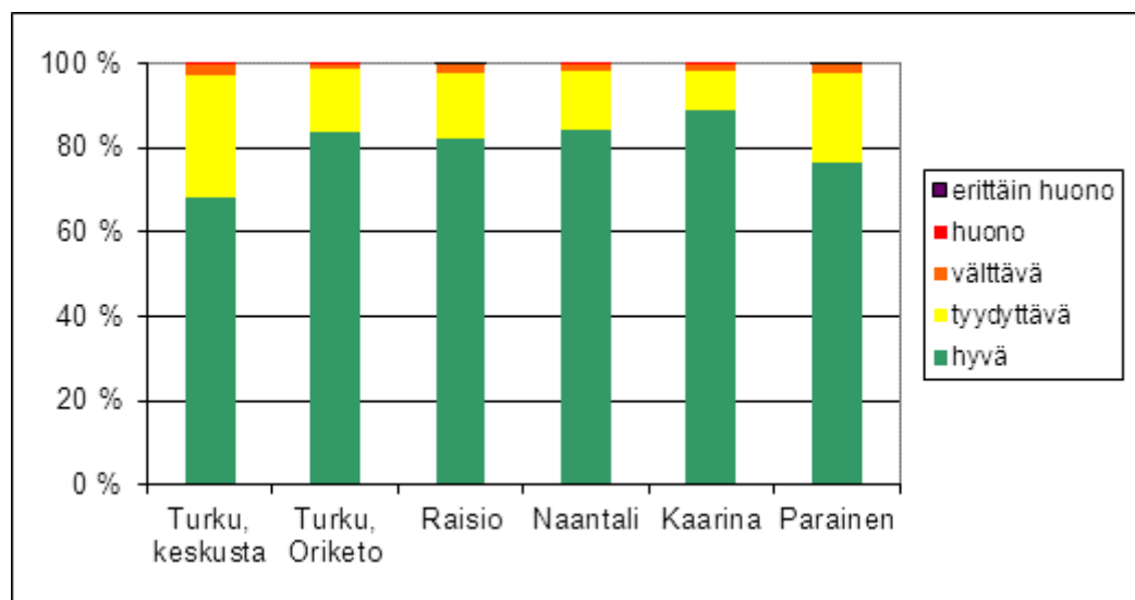
Kuva 6. Ilmanlaatuindeksin jakautuminen tunneittain eri luokkiin vuonna 2011.
