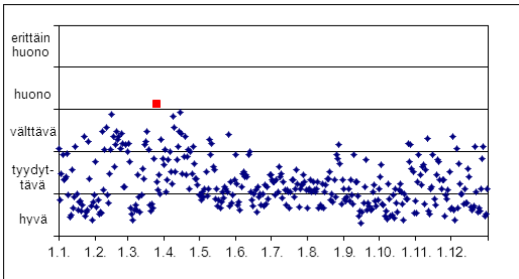
Kuva 40. Naantalin keskustan ilmanlaatu indeksillä kuvattuna vuonna 2011.
