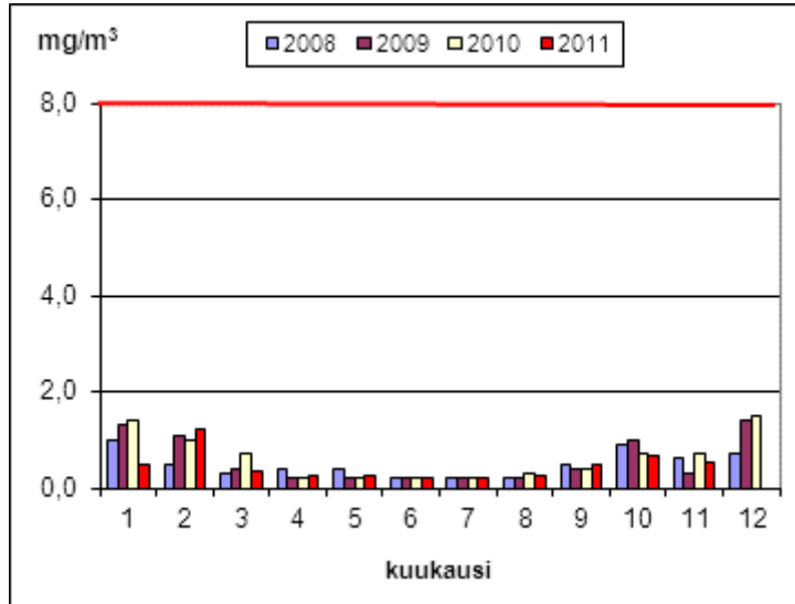
Kuva 24. Hiilimonoksidin ohjearvoon ( 8 \text{ mg/m}^3 ) verrattavat 8 tunnin keskiarvot Kauppatorilla vuosina 2008 - 2011. Joulukuun 2011 tulokset puuttuvat laitevian vuoksi.
