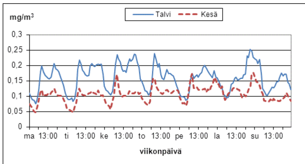
Kuva 25. Kauppatorin hiilimonoksidin pitoisuuden vaihtelut viikon eri ajankohtina kesällä (1.4.-30.9.) ja talvella (1.1.-31.3. ja 1.10.-31.12.) vuonna 2011.
