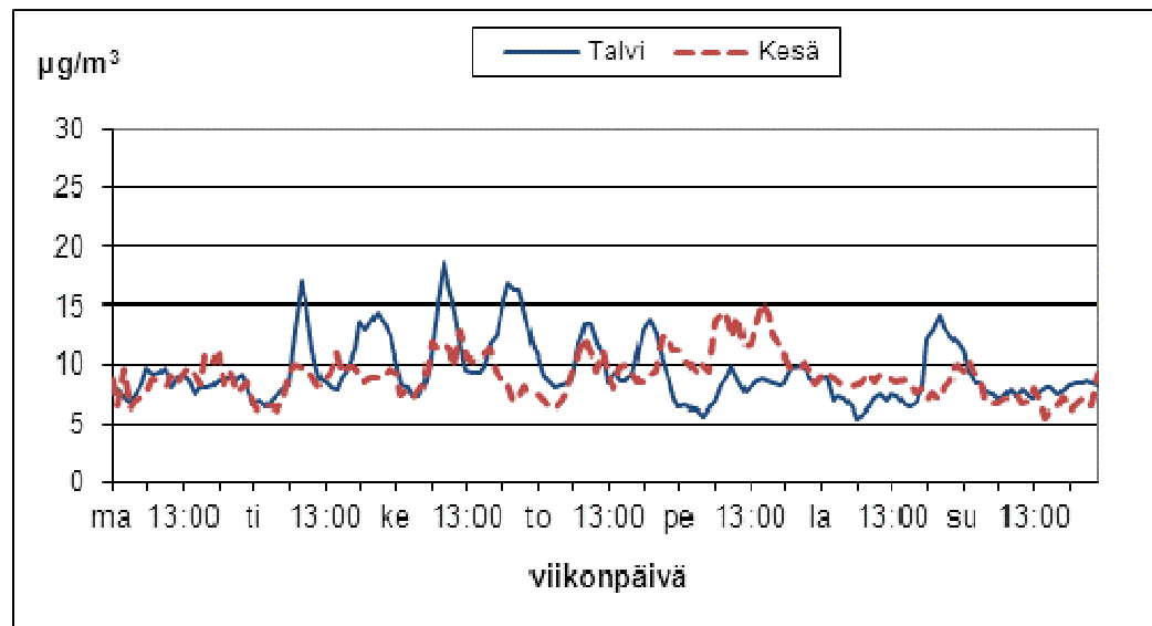
Kuva 57. Kaarinan hengitettävien hiukkasten pitoisuuksien vaihtelut viikon eri ajankohtina kesällä (1.4.–30.9.) ja talvella (1.1.–31.3. ja 1.10.–31.12.) vuonna 2011.
