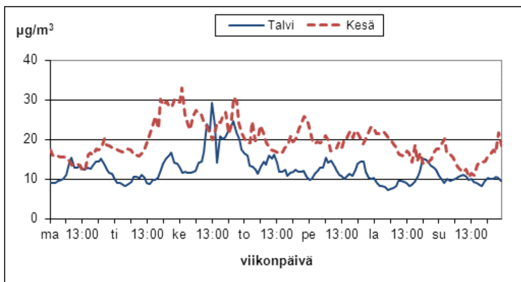
Kuva 60. Paraisten hengitettävien hiukkasten pitoisuuksien vaihtelut viikon eri ajankohtina kesällä (1.4.–30.9.) ja talvella (1.1.–31.3. ja 1.10.–31.12.) vuonna 2011.
